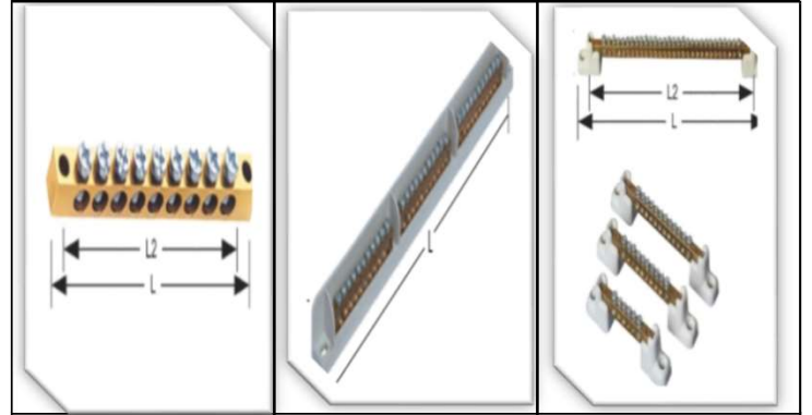
160 A.. 10x15mm 7-20 DEL.TOPRAK 3 KUTUPLU T.KL. 80 AMPER 80 AMP. 6,5x9mm 4-40 DEL NÖTR
