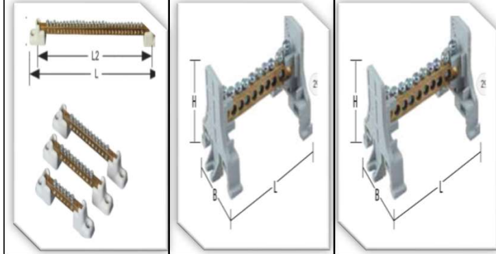
125 AMP. 7x12mm 4-40 DEL NÖTR 80 AMP. 6,5x9mm 7-30 DEL NÖTR 125 AMP. 7x12mm 7-30 DEL NÖTR
